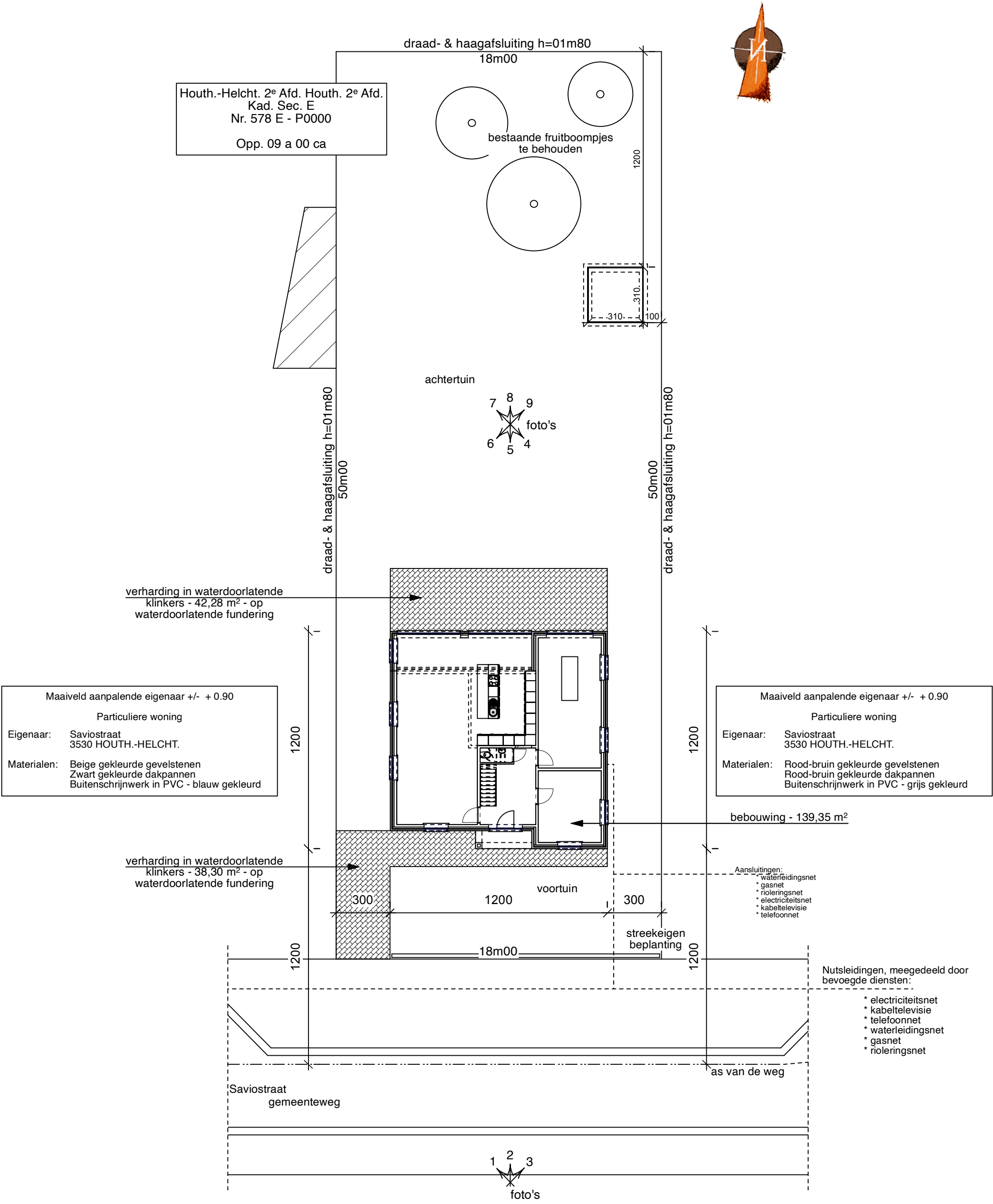
INPLANTINGSPLAN (schaal 1/200)
