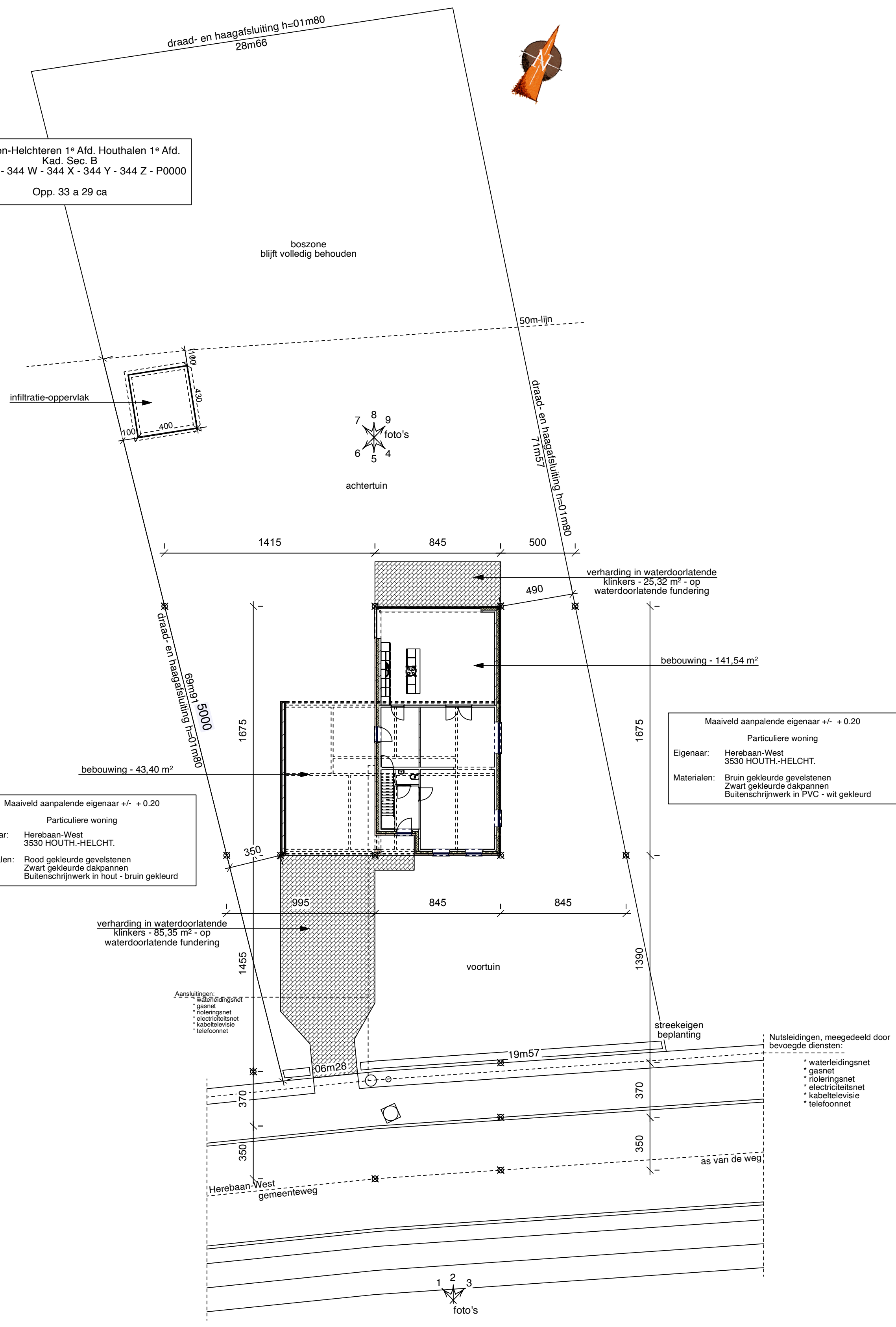
INPLANTINGSPLAN (schaal 1/200)
