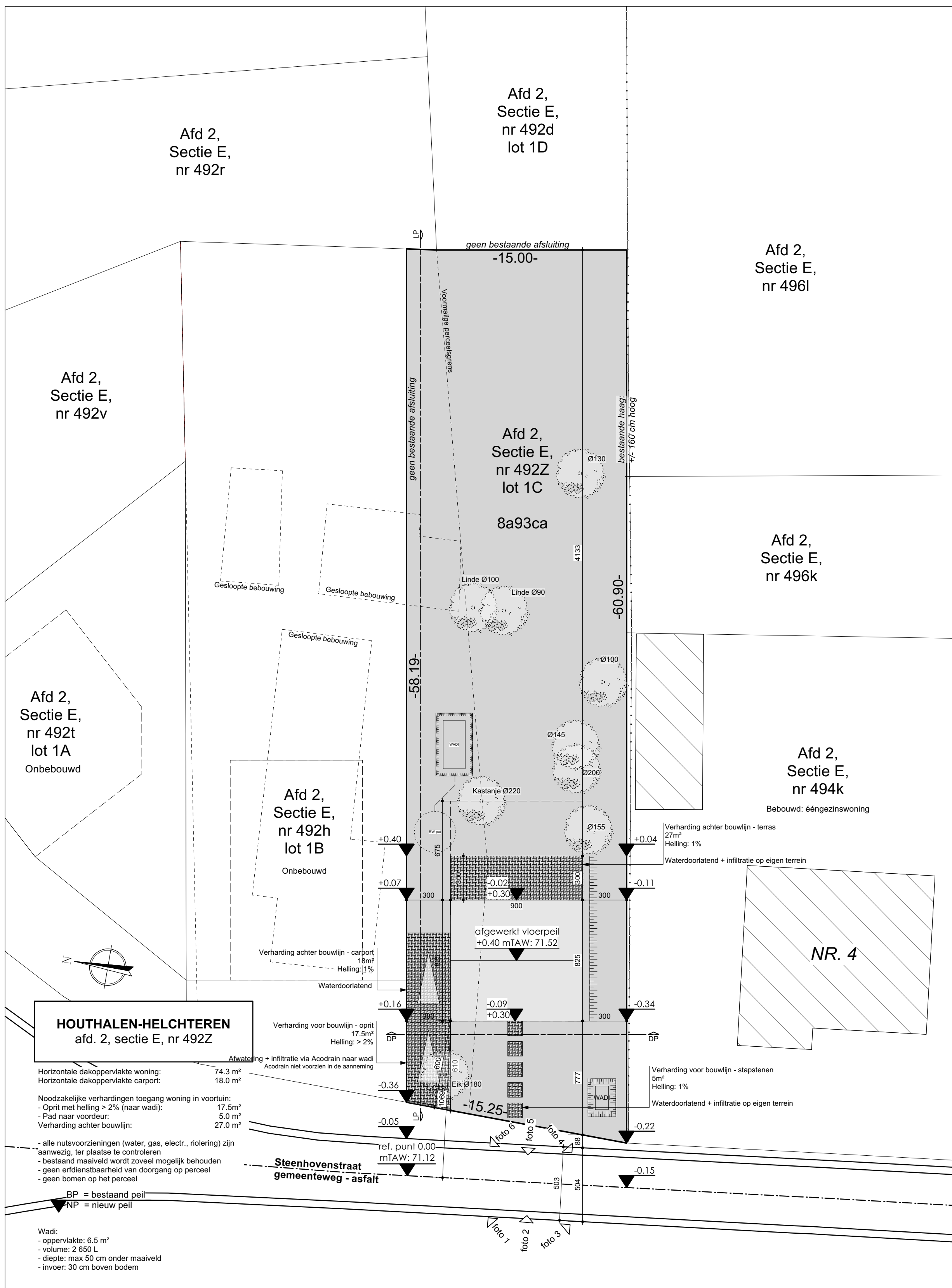
Inplantingsplan Schaal: 1:200
