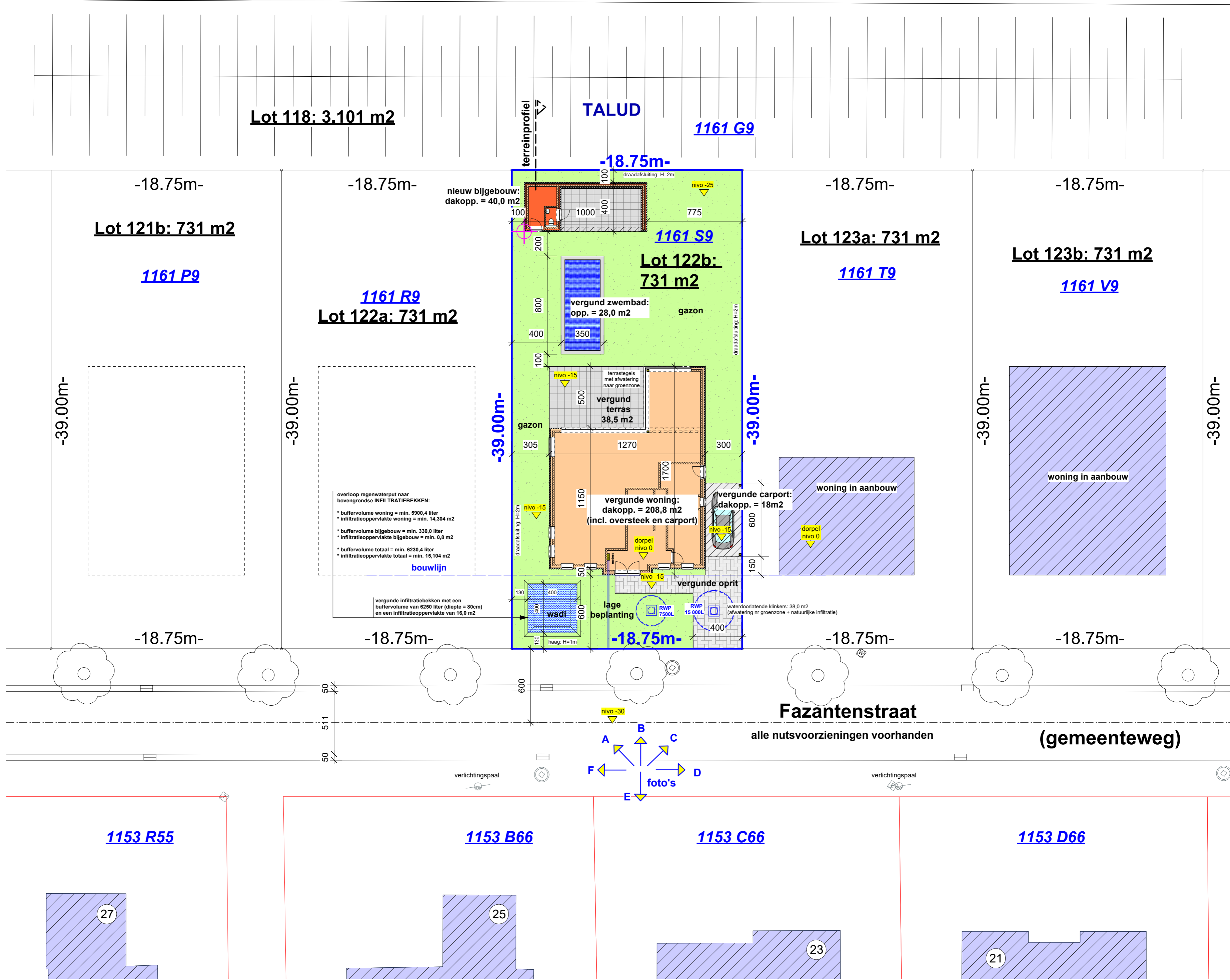
Inplantingsplan (schaal 1/200) gemeente Houthalen-Helchteren, Fazantenstraat LOT 122b
