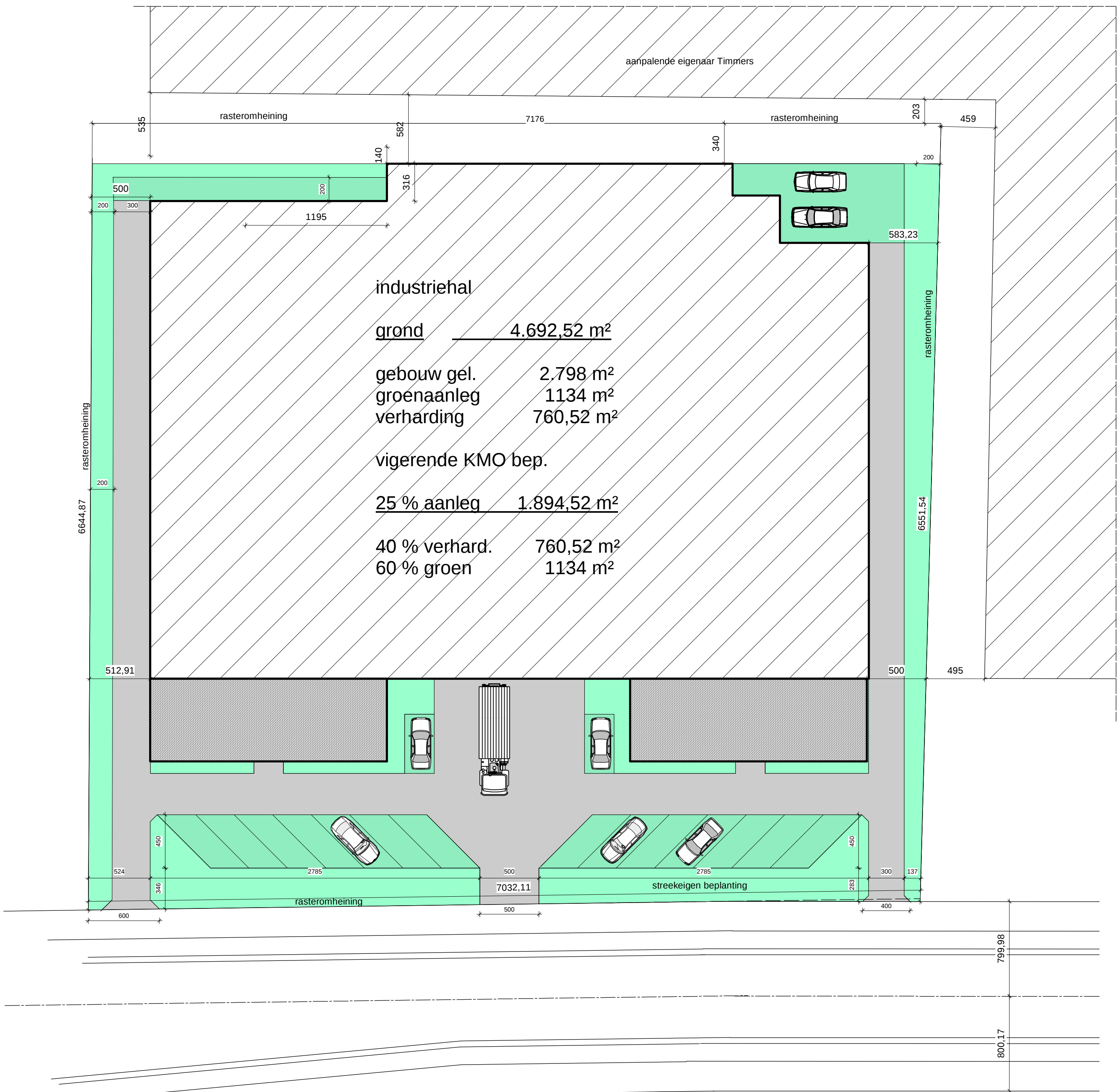
INPLANTINGSPAN sch. 1/250 - NIEUWE TOESTAND
