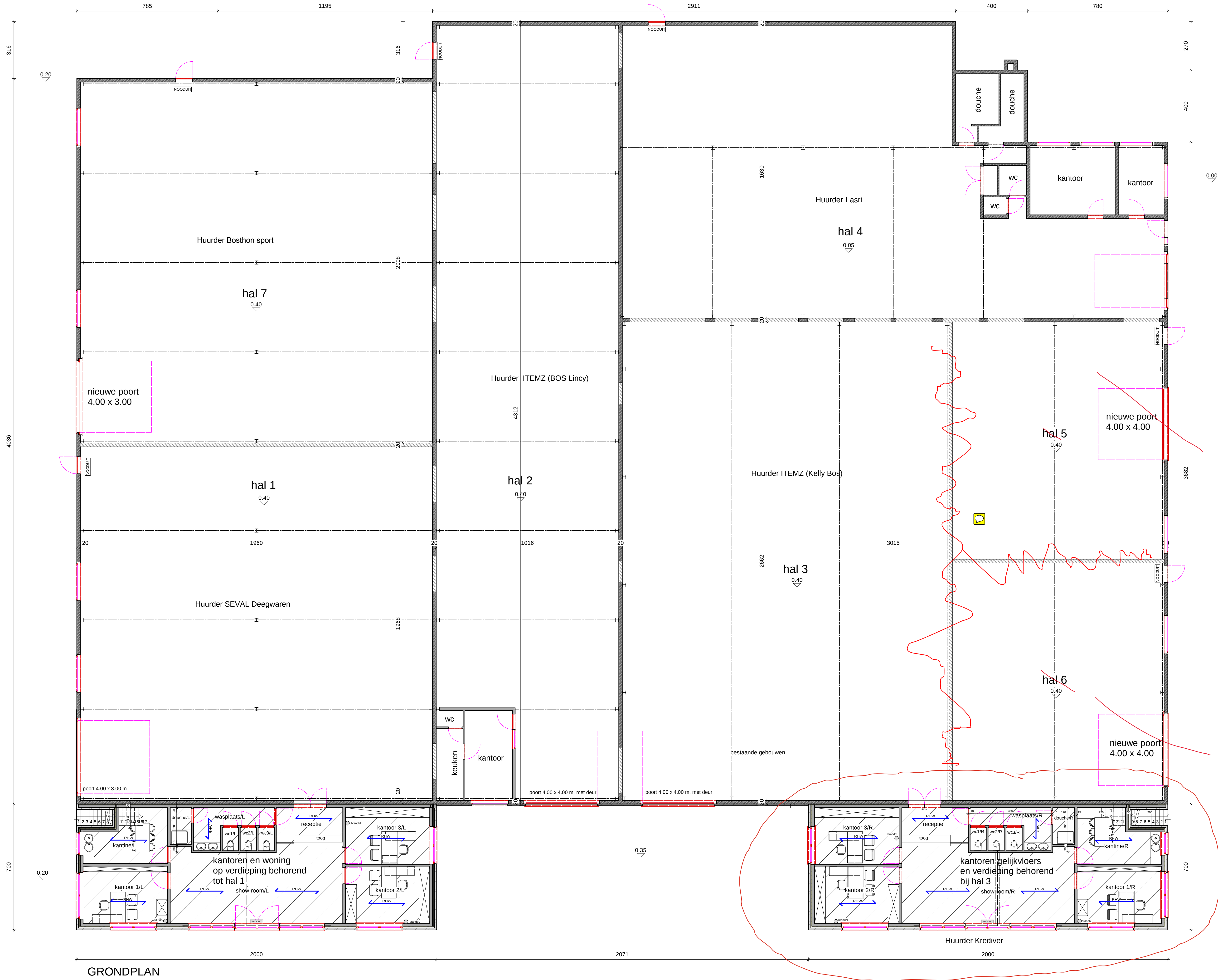
GRONDPLAN
