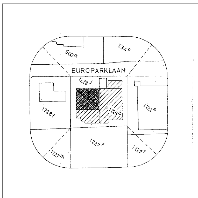
SITUERINGSPAN sch. 1/2.500
